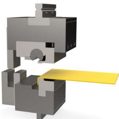
Speciaal gereedschap voor het produceren van een 90° buiging in horizontale positie
