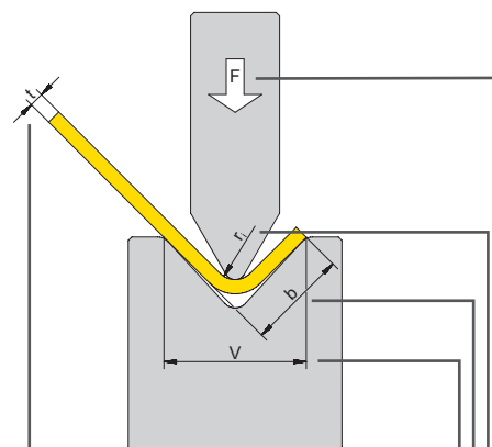
Perskrachttabel: Vereiste perskracht t.b.v. een 90° vrij- / luchtbuiging R m = 510 N/mm², staal
