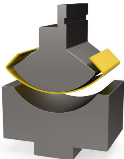
Radius doordrukgereedschap voor een grote radius met voorgekante beenlengte
