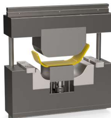
Gereedschap met stanggeleidingen en verende uitwipper, voor het kanten van een werkstuk met twee verschillende radii in één slag
