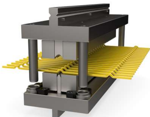
Meervoudig gereedschap voor het maken van golfvormen in rondmateriaal
