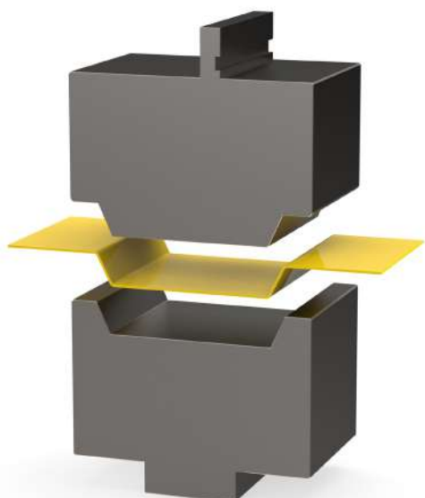
Trapezium buiggereedschap voor een groot trapeziumprofiel
