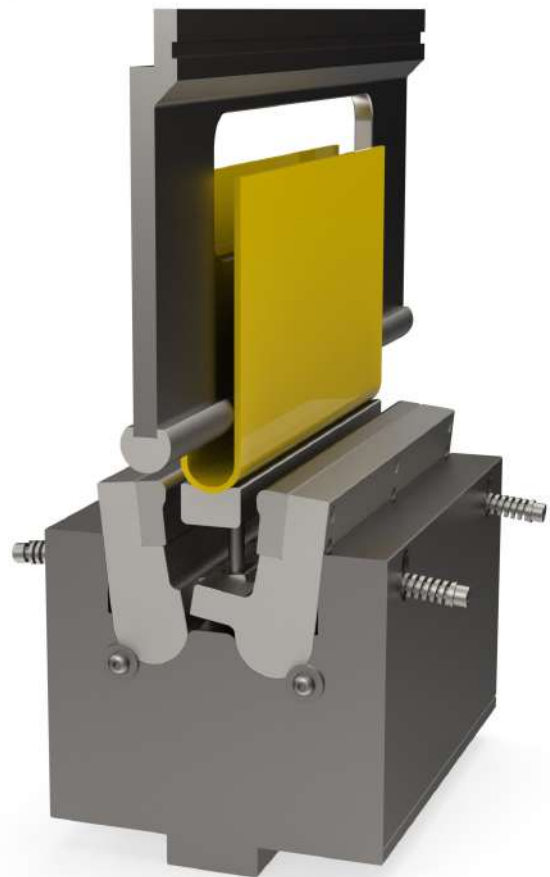
U-Buiggereedschap voor profielen met hoge benen
