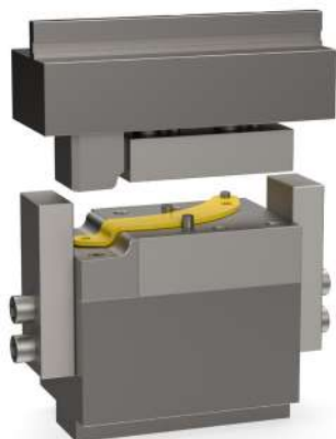
Station 1: Z-Drukgereedschap voor klemvorm, met veerbelaste neerhouder en zijdelingse steunen
