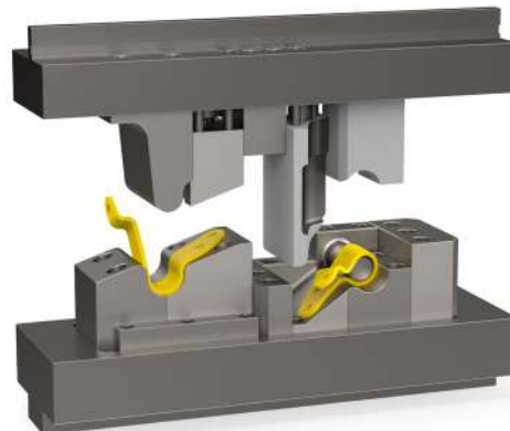
Station 2: Gereedschap voor het drukken van een radius (links) en het omrollen tot een klemvorm (rechts), met veerbelaste neerhouders en geïntegreerde steunen
