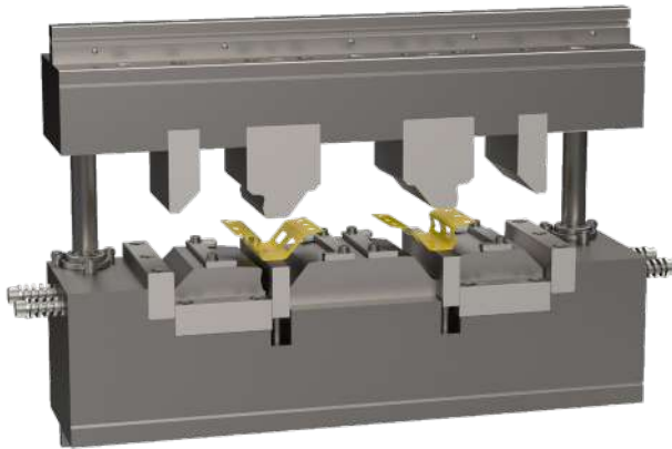
Meervoudig gereedschap
