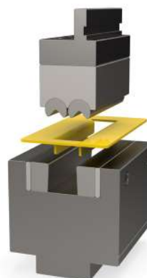
Speciaal gereedschap met beweegbare buiglijsten voor het produceren van twee inwendige 90° buigingen in een slag
