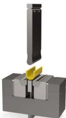
U-Buig gereedschap met beweegbare buiglijsten en uitwerper
