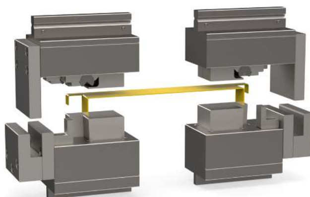
Vormgereedschap met veerbelaste neerhouders en draaibare wangen, voor het maken van vier 90° buigingen in één slag
