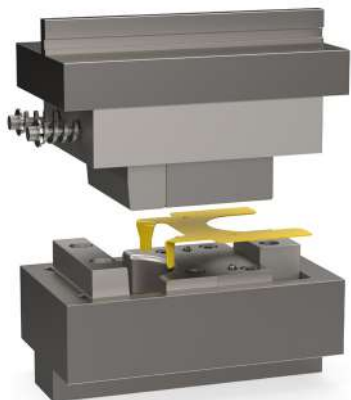
Station 1: Drukgereedschap voor twee 90° benen met een 3D-vorm
