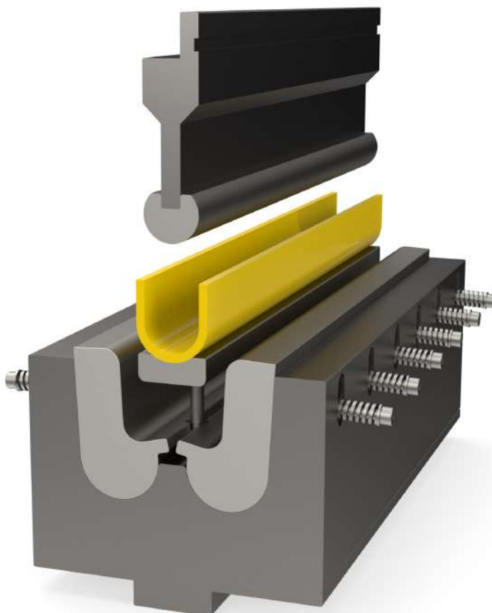
U-Buiggereedschap met beweegbare doorbuiglijsten
