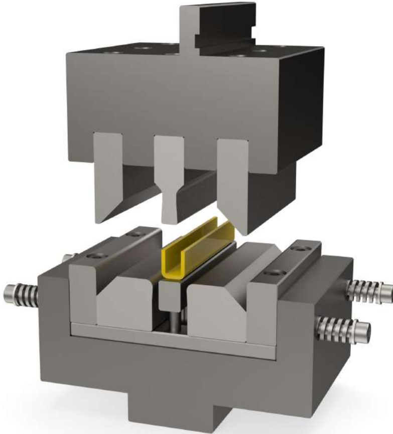
U-Buiggereedschap met spie-wig techniek om de terugvering van het materiaal te compenseren
