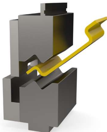
Z-Buiggereedschap met achtergeleider voor dik materiaal
