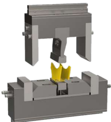
U-Buiggereedschap met spie-wig techniek voor een asymmetrische U-vorm
