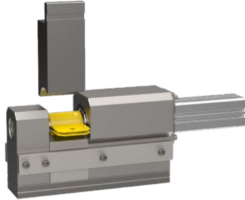
Station 2: Sluiten van het klemprofiel. Gereedschap met pneumatisch gestuurde buigdoorn voor geautomatiseerde uitname
