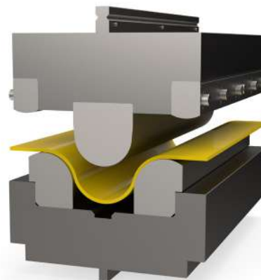
Rondvorm gereedschap met instelbare buiglijsten
