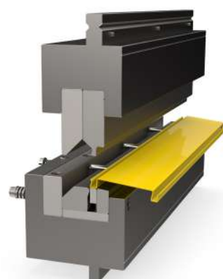
U-Buig gereedschap met spie-wig techniek voor profielen met aanliggende 90° buiging
