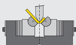
V-buigen
