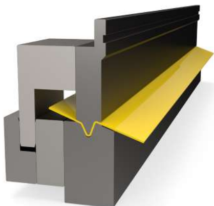
Drukgereedschap met ruggeleiding voor asymmetrische V-vormen
