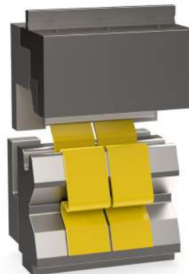
Station 2: V-Drukgereedschap met ruggeleiding aangepast aan de eerste U-buiging
