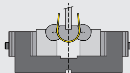
Radius-buigen / overbuigen
