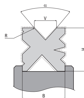
Opname Multi-V ondergereedschap
