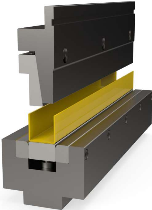
U-Buiggereedschap met verend bovendee voor een proces zekere uitname
