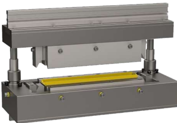
Speciaal gereedschap met spie-wig techniek voor meerzijdige buiging
