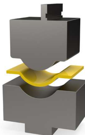
Gereedschap voor een grote ronde versteving
